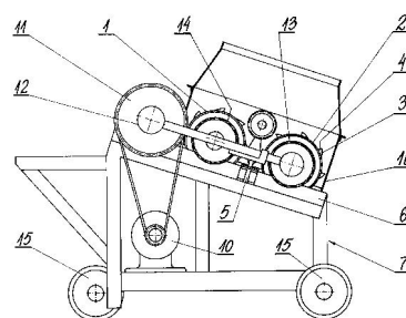
rys. urządzenie do rozdrabniania odpadów
